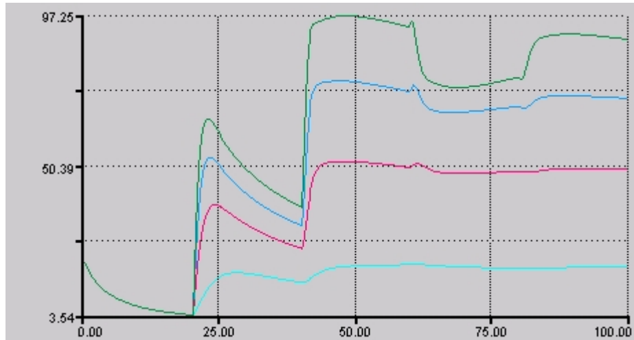
Figura 7: Evolución temporal de la variable No susceptibles 2 del sistema de protección. Cada gráfica corresponde a un valor del parámetro PROTMAX (0.1, 0.4, 0.7 y 1)
